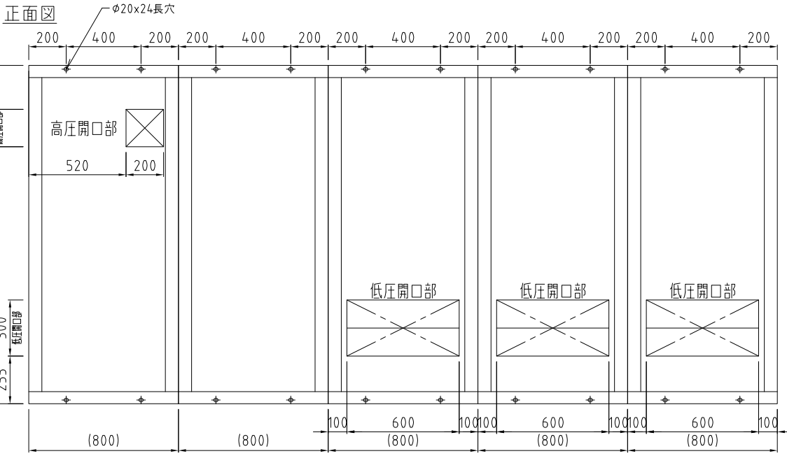
ベース上面図 (A-A断面図)
