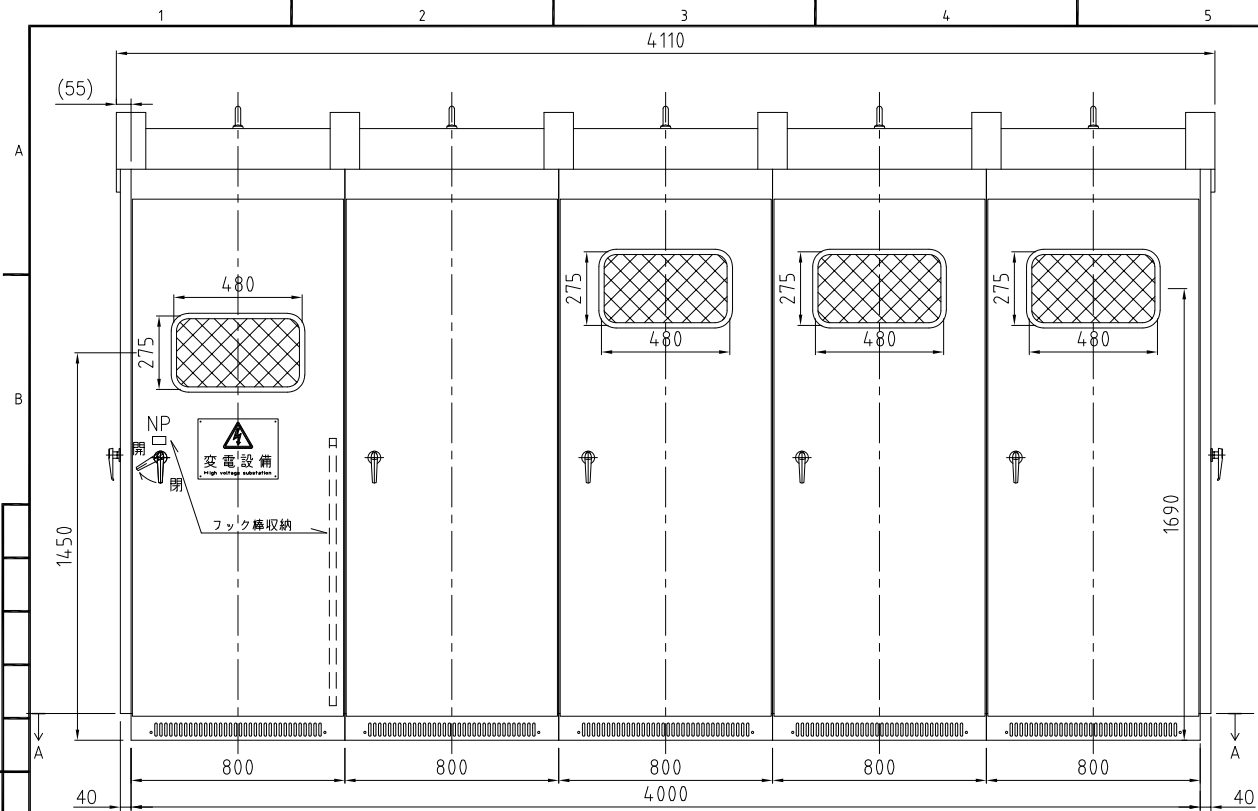
正面図
