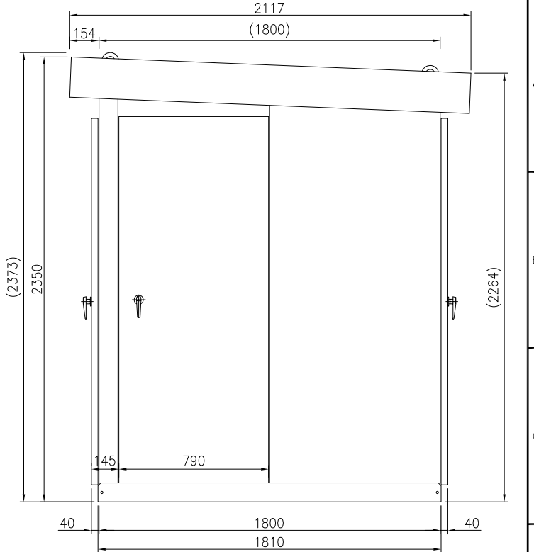
右側面図
