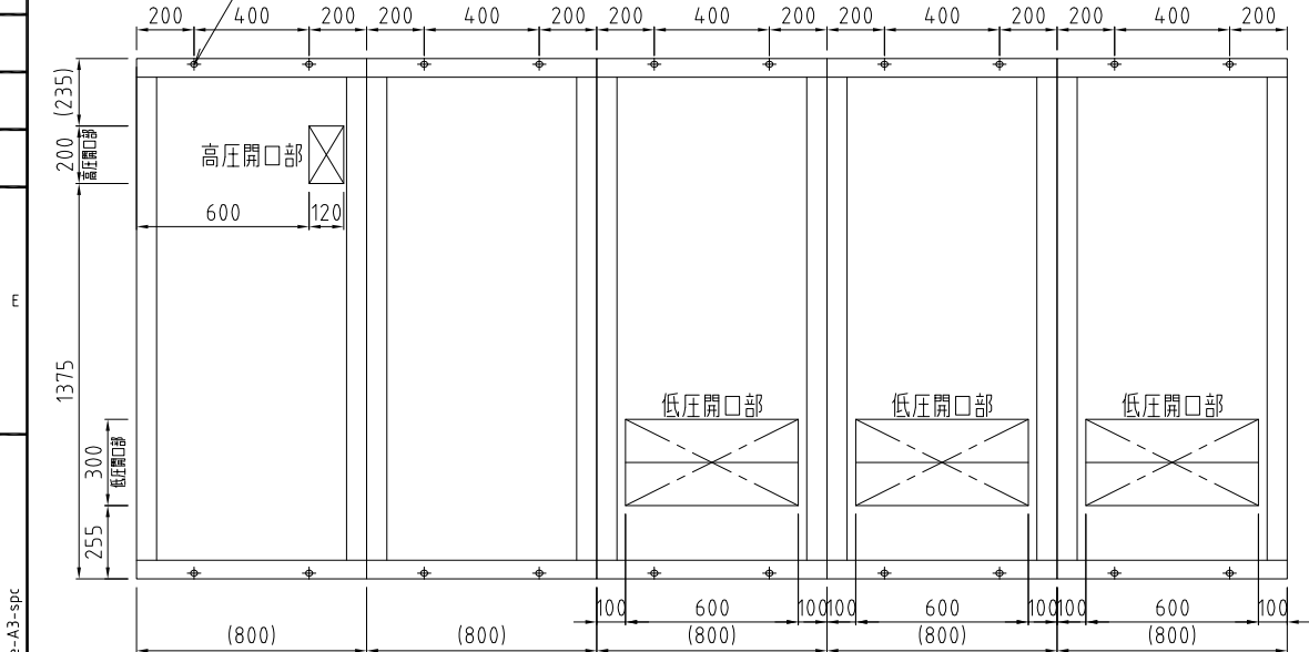
ベース上面図 (A-A断面図)
